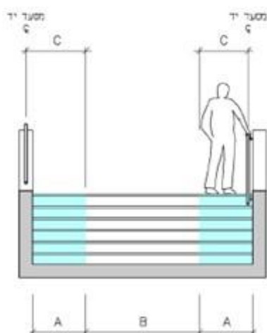
כאשר A – תחום רוחב המדרגה הנדרש למילוט B – תחום רוחב המדרגה שאינו נדרש למילוט אז C – המרחק אל בית האחיזה 0.75 \geq C מטר
