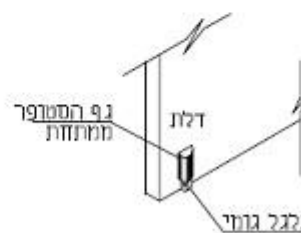
פרט 10 חלק תחתון של הדלת
