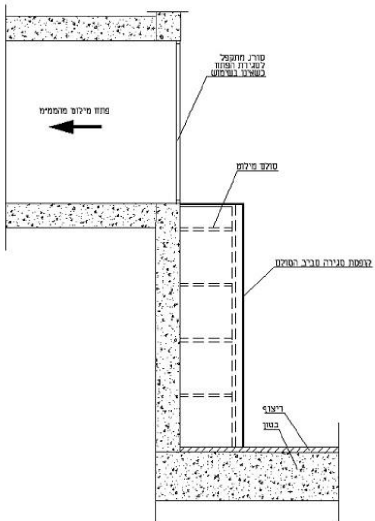
פרט 4 סגירת סולם מילוט, חתך א-א' קני"מ 1:10
