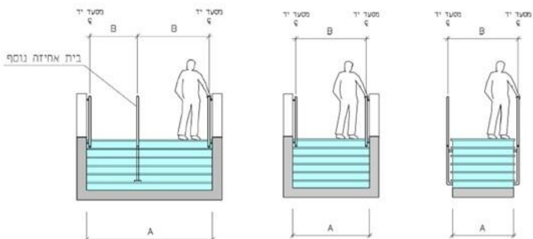
כאשר A – תחום רוחב המדרגה הנדרש למילוט אז B – המרחק בין בתי האחיזה 1.50 \geq B מטר
